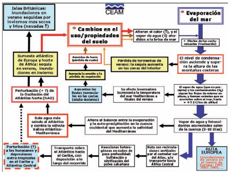
Figura 15.- Retro-alimentaciones entre los cambios de uso del suelo en la Cuenca Mediterránea Occidental y el sistema climático-hidrológico (Millán; en EC 2007). En esta figura el camino del vapor de agua está señalado con flechas azules, los efectos directos con flechas negras, y los efectos indirectos con otros colores. Los umbrales críticos, remarcados en rojo, indican cuando el sistema puede caer a un nuevo estado.
