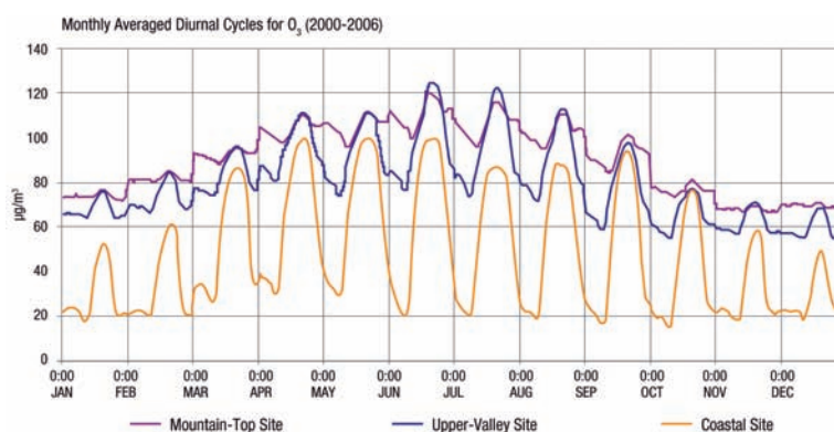
Figura 11.- Evolución anual de los ciclos diurnos (promediados mensualmente) en las estaciones indicadas durante los años 1997-2002. Los ciclos diurnos de O 3 en las estaciones en línea de costa (GRAO) muestran su mínimo absoluto a primeras horas de la mañana (Figuras 1, 8) cuando aumenta el tráfico (emisiones de NO x ), y el viento aún sopla desde tierra. Los extremos en este tipo de estación muestran un primer máximo en abril-mayo (primavera), y otro máximo de los máximos en septiembre (distribución en forma de M). En las estaciones situadas dentro de la zona de regeneración (o producción) de O 3 , (Tipos #2), Upper Valley (#3) y/o Tipo # 4 (Mountain top), muestran sus máximos en junio-agosto. En este ejemplo, en Vilafranca (VILA) y Corachar (CORA). La diferencia entre el máximo en la estación costera y el de dichas estaciones representa la producción fotoquímica adicional, que producen las emisiones (locales) en la costa, sobre los niveles que entran con la brisa. Y, estos proceden del fondo regional resultante de las recirculaciones verticales de los días previos. Los niveles promedio de este fondo son \approx 90 \mu\text{g}/\text{m}^3 . Esta situación deja muy poco margen (solo unos 30 \mu\text{g}/\text{m}^3 ) para cualquier tipo de actuación de control local, y presenta muchos problemas a la hora de elaborar planes de actuación (sobre las emisiones locales) o, simplemente, si hay que informar al público, o dar alertas a la población.
